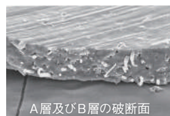
A層及びB層の破断面
